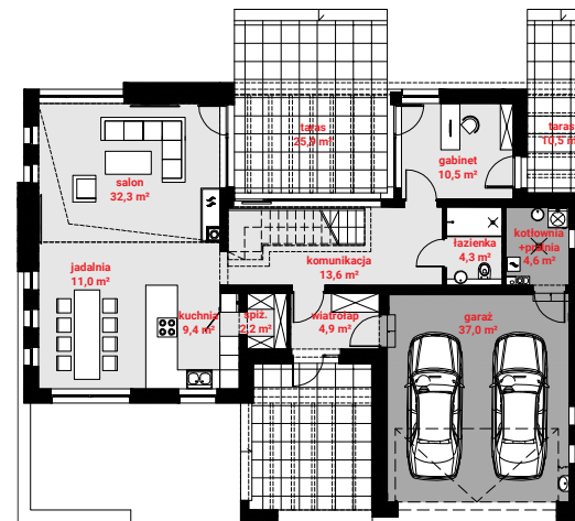
Parter: pow. użytkowa 92,7 + garaż 37 m 2
