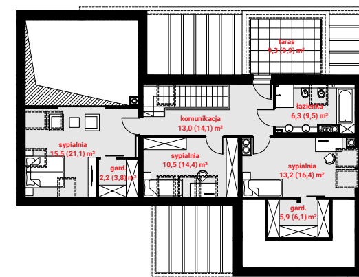
Poddasze: pow. użytkowa 66,6 (pow. podłóg 85,2) m 2
