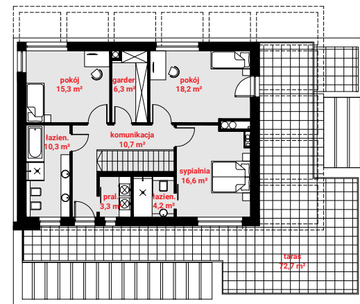
Piętro: pow. użytkowa 84,9 m 2
