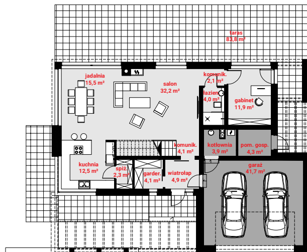
Parter: pow. użytkowa 101,7 + garaż 41,7 m 2
