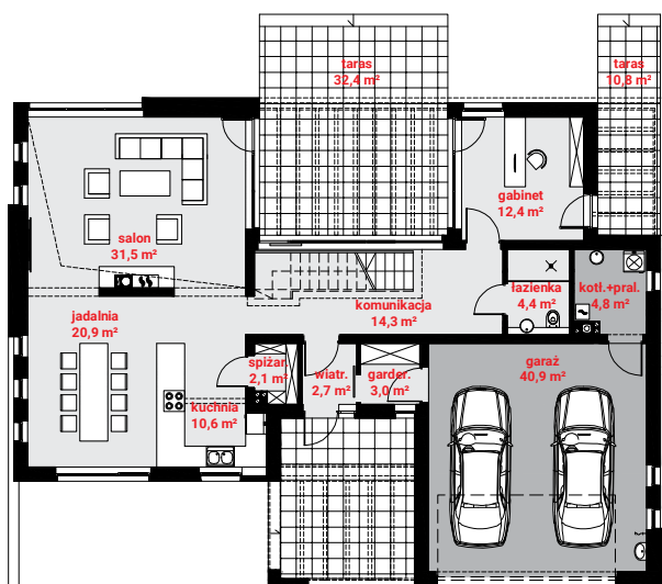
Parter: pow. użytkowa 106,7 + garaż 40,9 m 2
